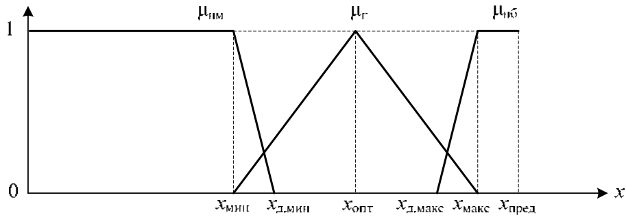
Рис. 3. Функции принадлежности нечетких переменных \mu_{нм} («не годен меньше»), \mu_г («годен»), \mu_{нб} («не годен больше»)
